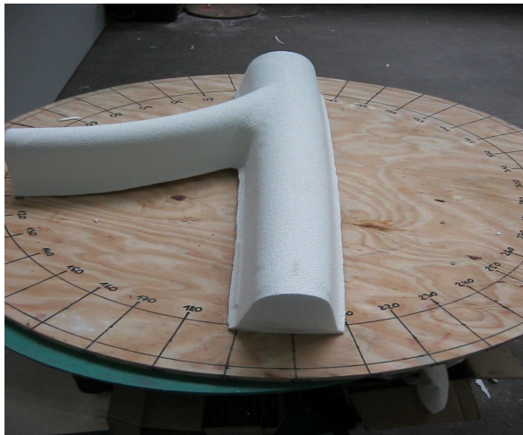
Winkelkontrolle des Gerinnenegativ mit Seitenzulauf
