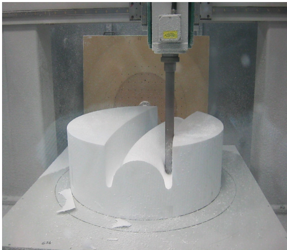
Software gesteuerte, automatische Gerinneformbearbeitung im Fräszentrum
