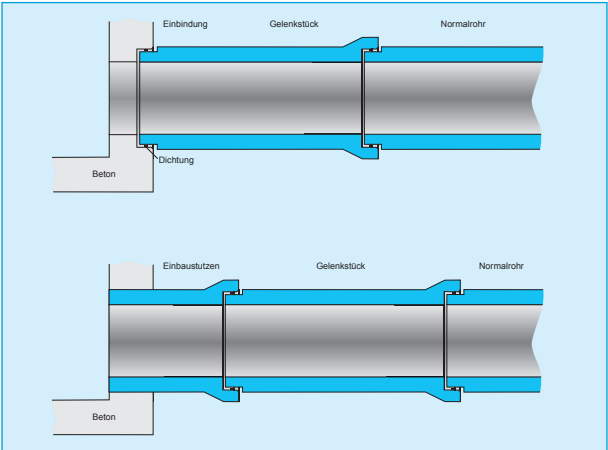
Bild 11: Mögliche Varianten eines Rohranschlusses an ein Bauwerk
